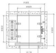
井道平面布置图 (旁开双开门)
